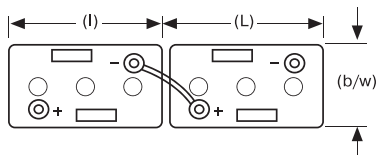
OPzS Solar 190-1080
