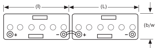
OPzS Solar 3100-3350
