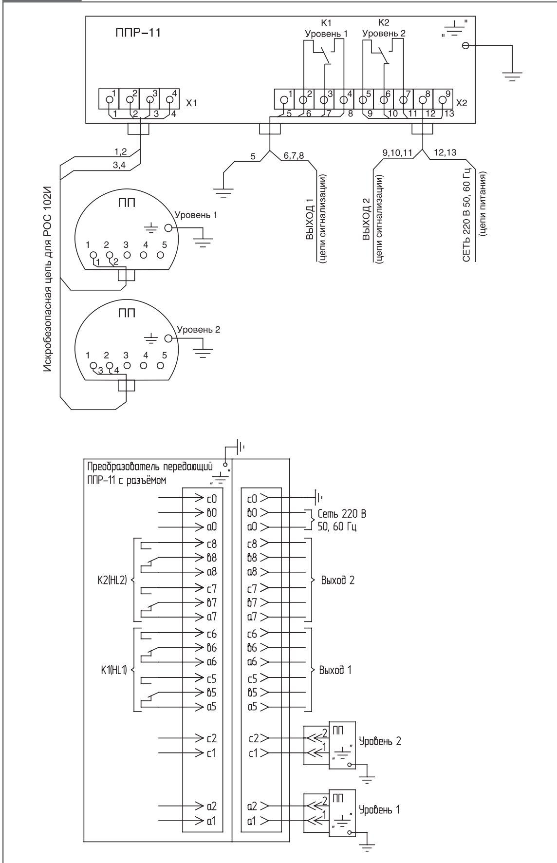
Схема электрическая подключения РОС 102И.
