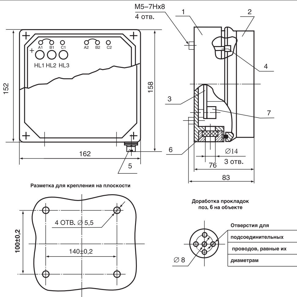
Габаритные размеры передающего преобразователя с разъемом.
