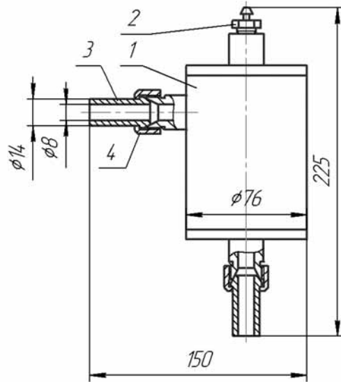
Сосуды уравнивающие СУ-40.
