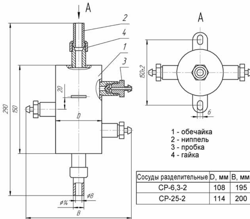
Сосуды разделительные исполнения 2 СР-6,3-2; СР-25-2.
